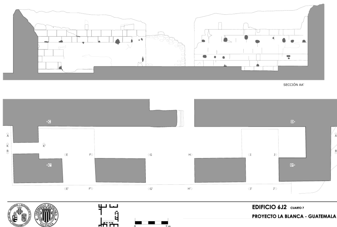
Figura 3 Planta y sección del Cuarto 7 del palacio 6J2 (Levantamiento G. Muñoz Cosme, A. Peiró Vitoria, Z. Herguido Alamar, V. De Anchel Benlliure y P. Díaz Rodríguez).
