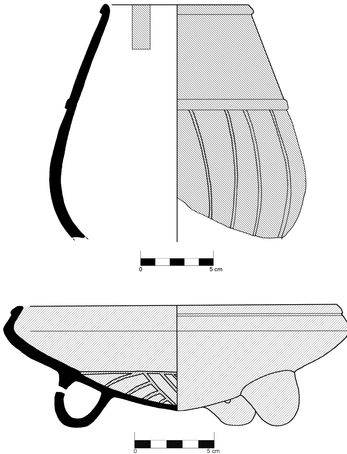
Figura 6 A y B. Recipientes cerámicos del Clásico Terminal, pertenecientes a la Clase Petén Lustroso (a) y Naranja Fino (b) (Dibujo P. Morales).
