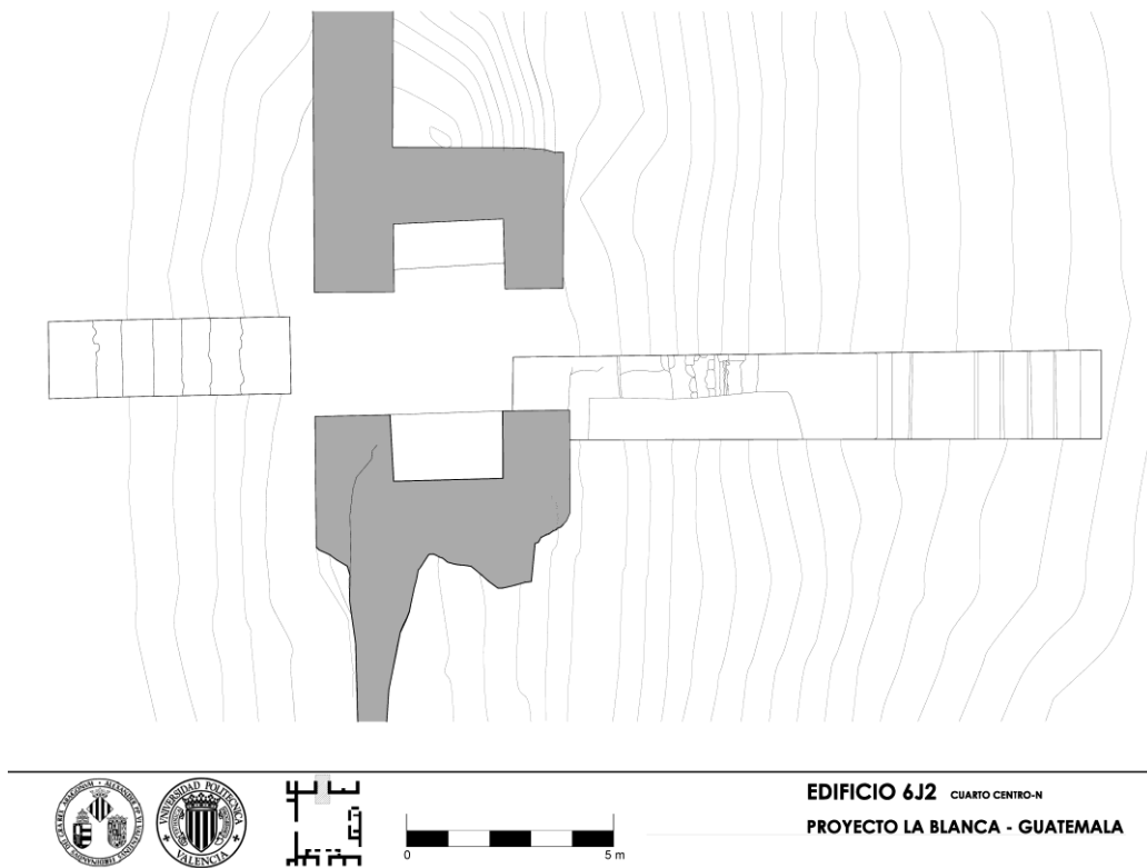
Figura 4 Planta del cuarto central del Sector Norte de la Acrópolis (Levantamiento G. Muñoz Cosme, A. Peiró Vitoria, Z. Herguido Alamar, V. De Anchel Benlliure y P. Díaz Rodríguez).
