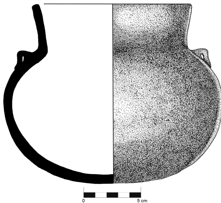
Figura 5 Olla de cerámica del Postclásico Temprano hallada en el derrumbe del cuarto central del Sector Norte de la Acrópolis (Dibujo P. Morales).
